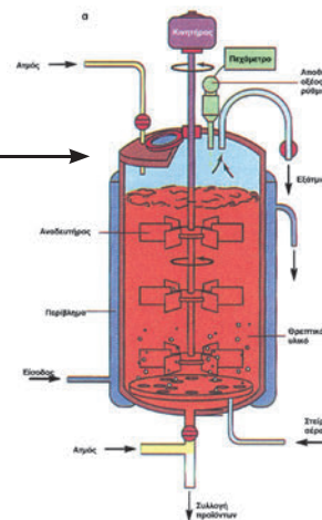
Εικόνα 7.3 α. Διαγραμματική απεικόνιση βιοαντιδραστήρα, όπου φαίνονται τα διάφορα τμήματά του, καθώς και οι συσκευασίες ελέγχου των συνθηκών ζύμωσης β. Φωτογραφία βιοαντιδραστήρα.
